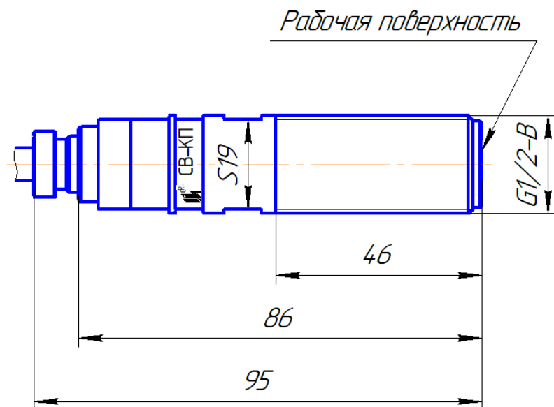
Рисунок А.6 - Габаритно-монтажный чертеж СВ-КП
