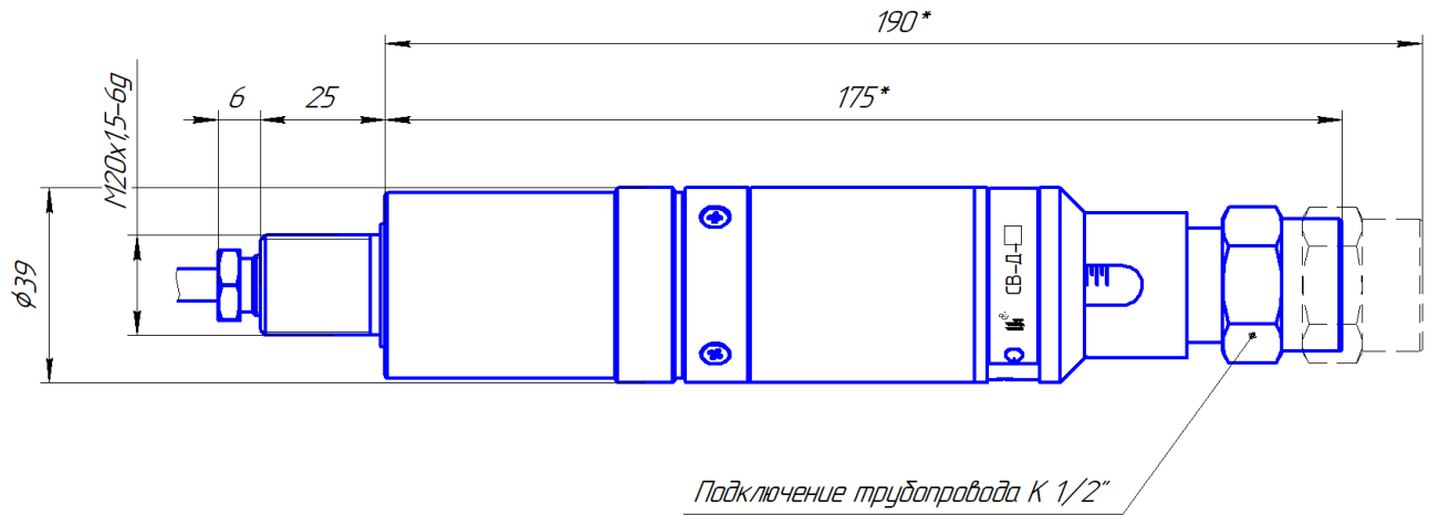
Рисунок А.4 - Габаритно-монтажный чертеж СВ-Д
