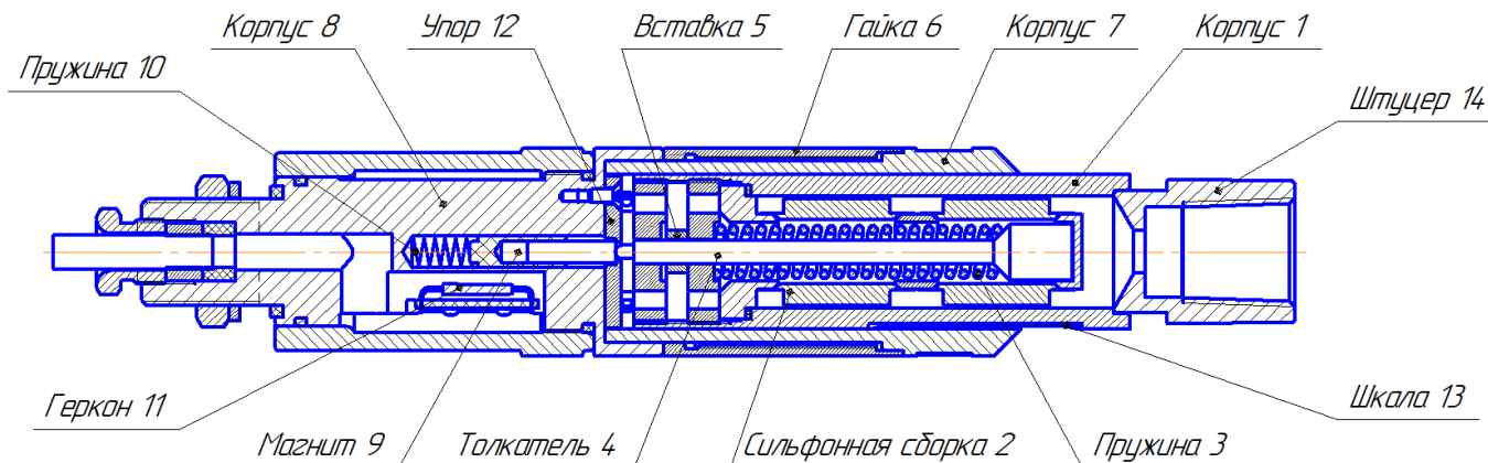
Рисунок 4.3 - Конструкция СВ-Д
