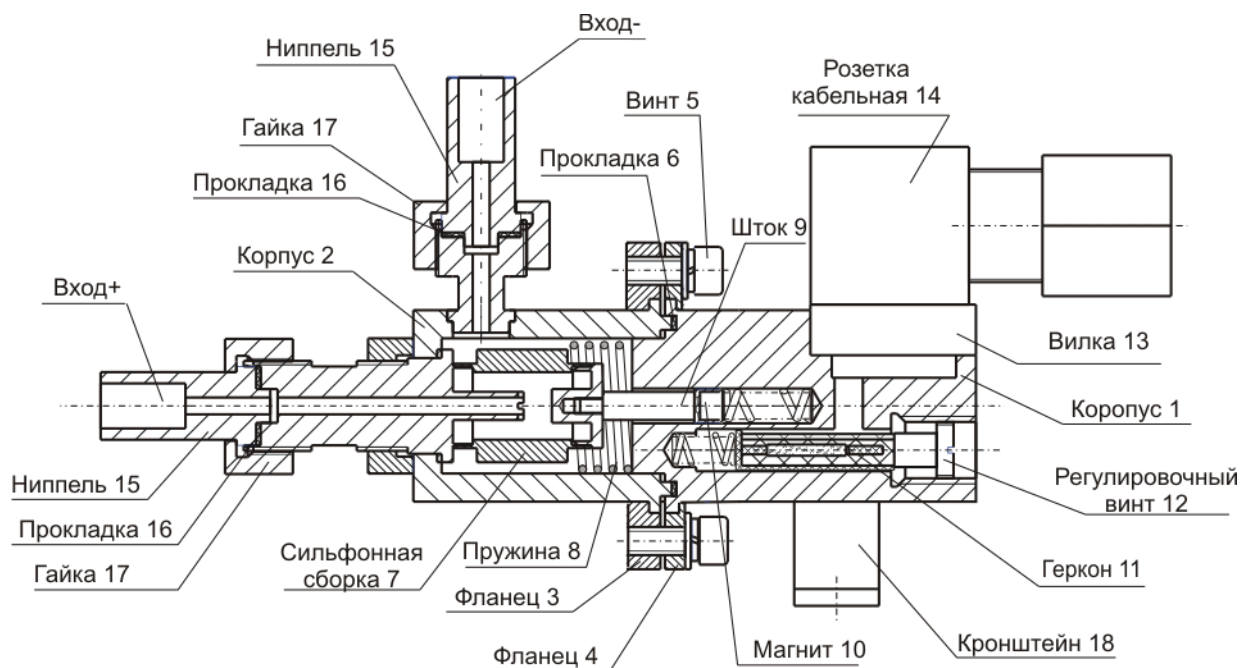
Рисунок 4.4 - Конструкция СВ-ДД
